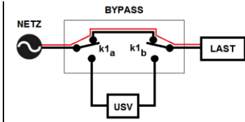
Abb. 15-3 Bypass-Betrieb
