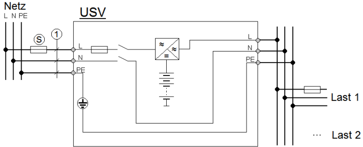
Abb. 5-2 Anschlussschema der USV an das Netz und die Verbraucher.
