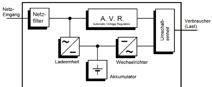
Abb. 3-1 Blockbild bzw. Aufbau der OFFICE-RM-Serie.
