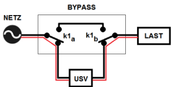
Abb. 15-2 USV-Betrieb
