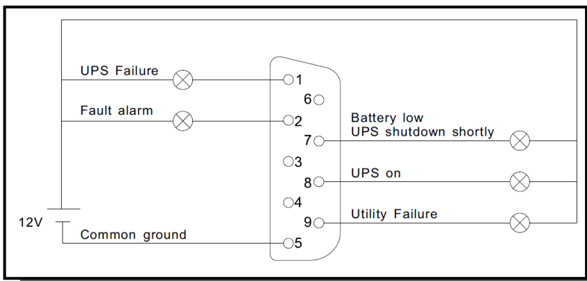
Abb. 3-2 - 4 Belegungsplan Relais-Karte (24V/1A)
