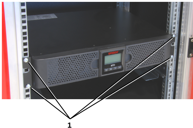
Abb. 3-3 - 9 Befestigung der USV im 19" Rack
