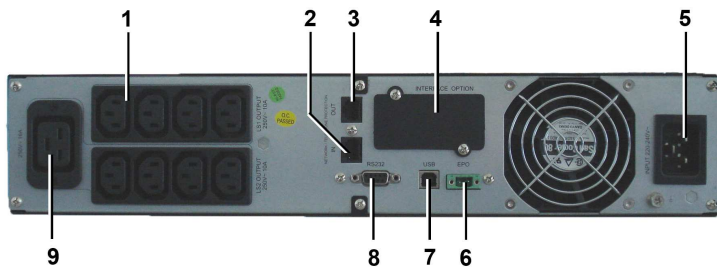
Abb. 3-2 - 1 Rückwand-Ansicht MTD-XL 2000
